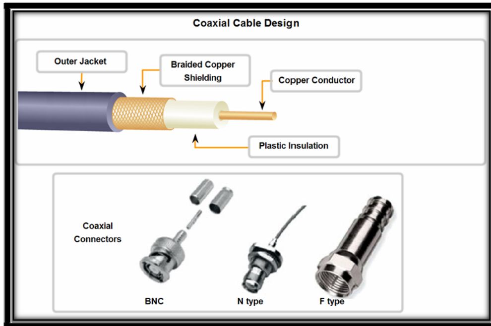
Gambar 1.12 Kabel koaksial
