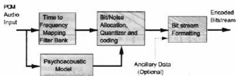
MPEG/Audio encoder
