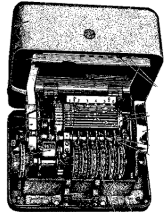
Enigma Rotor Machine
