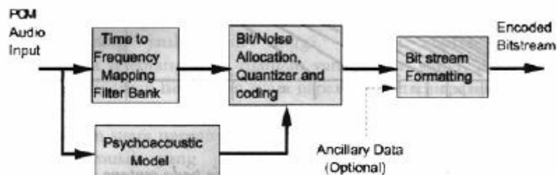
MPEG/Audio encoder
