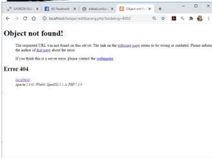
Gambar 13.2. Error Editbarang
