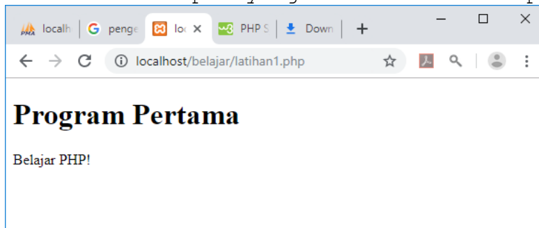
Gambar 2.1.Hasil Latihan1.php
