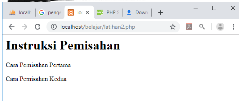
Gambar 2.2. Pemisahan Instruksi
