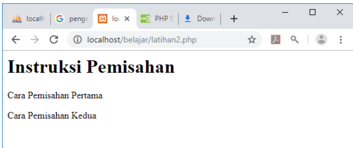
Gambar 10.2. Pemisahan Instruksi
