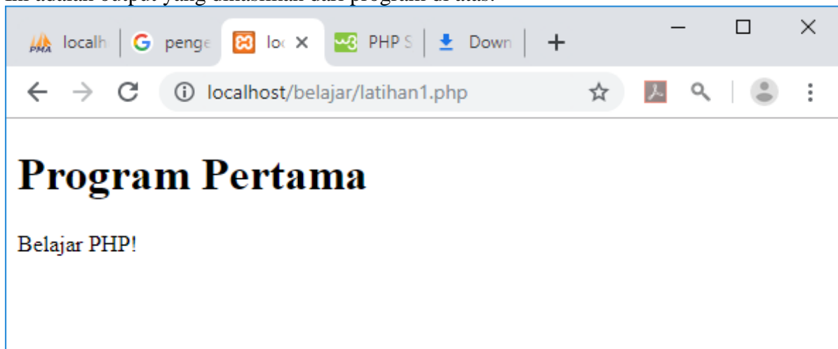
Gambar 10.1. Hasil Latihan1.php
