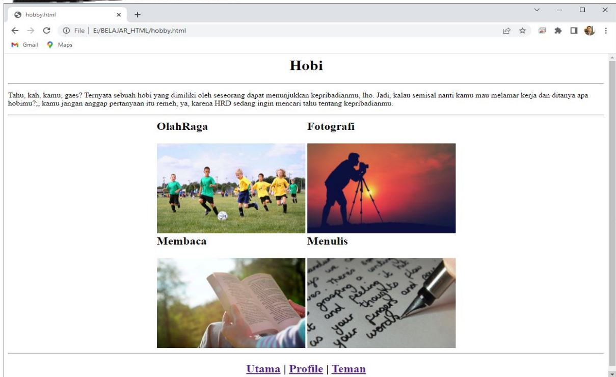
Gambar 6.10. Halaman Hoby.html
