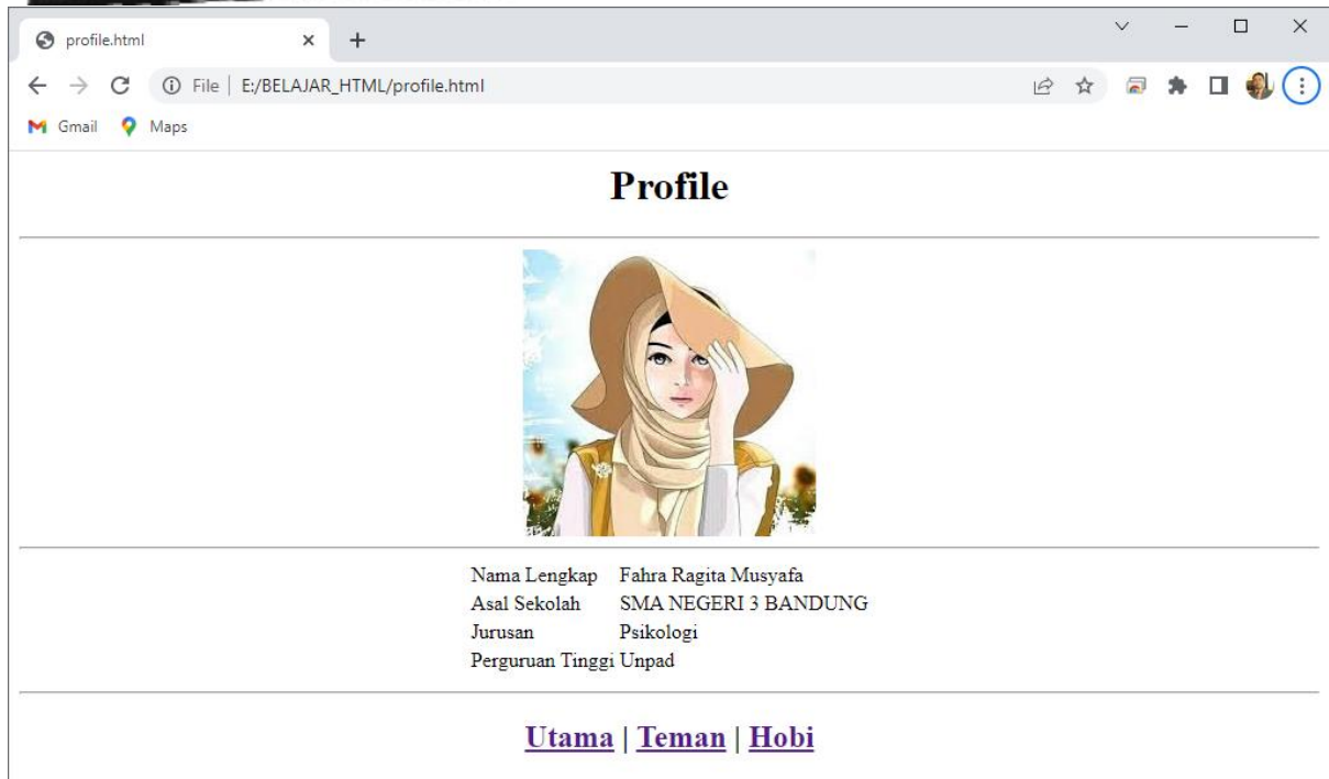
Gambar 6.8. Halaman profile.html
