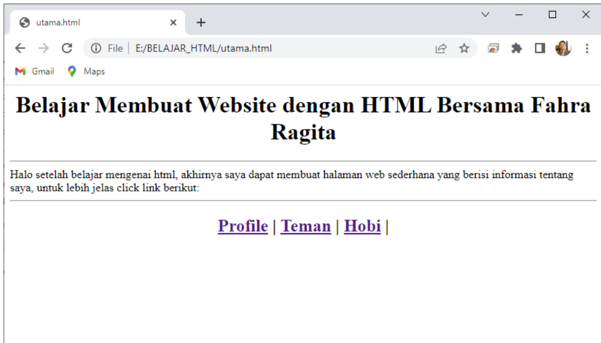
Gambar 6.7. Halaman utama.html
