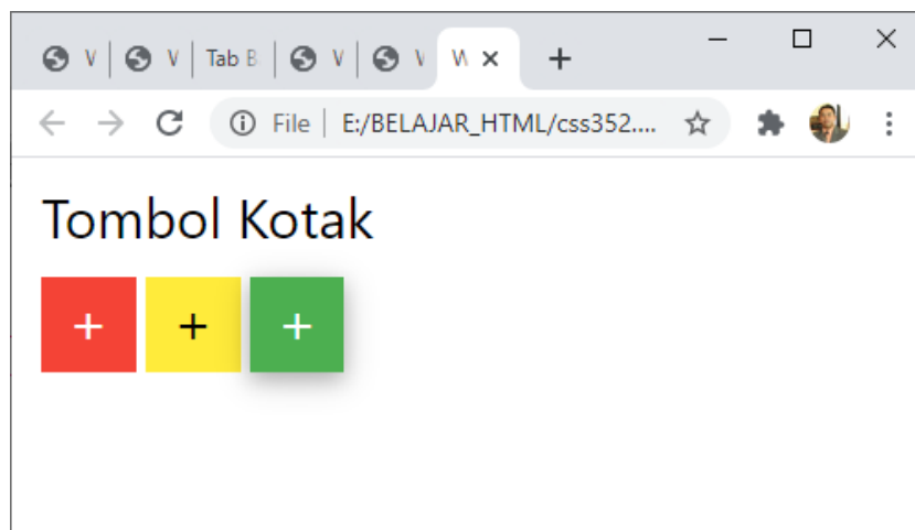
Gambar 10:12 Tombol Kotak
