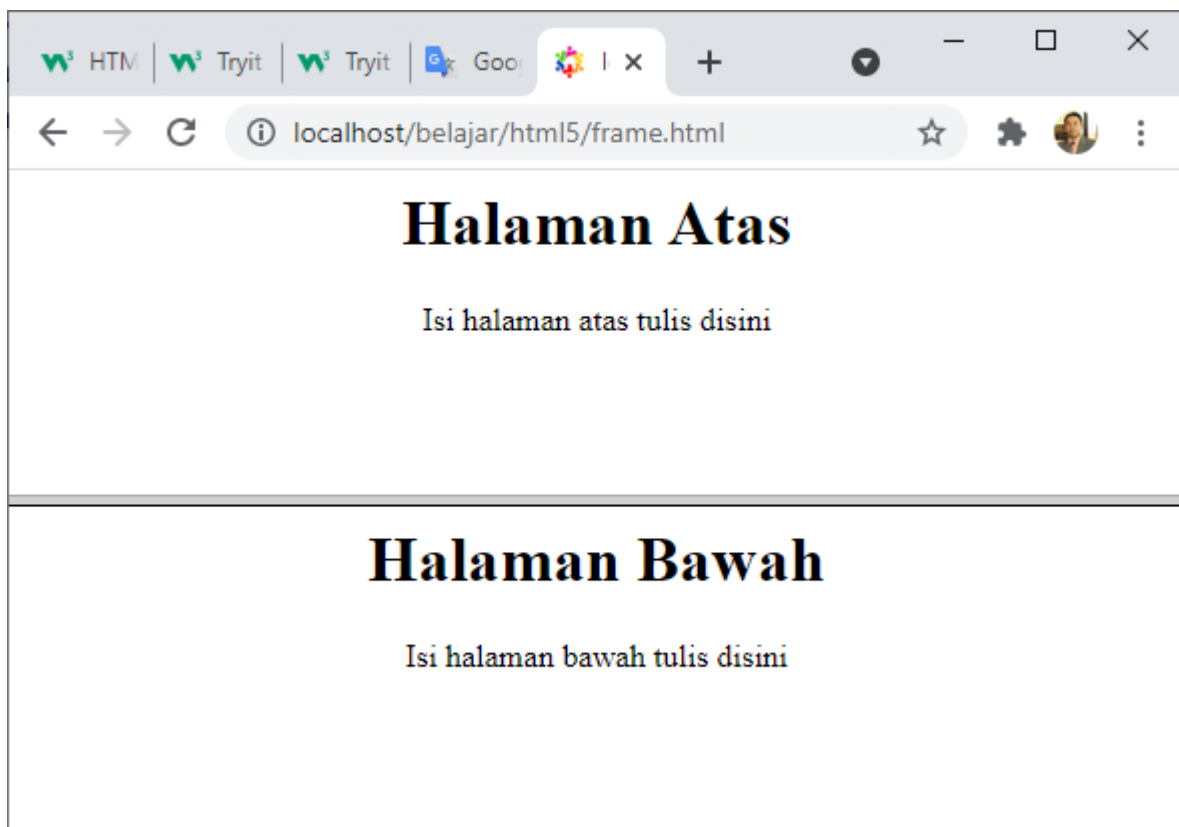
Gambar 7.1. Frameset 2 Baris
