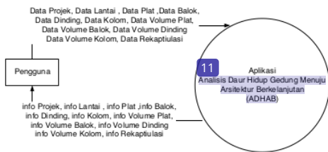
Gambar 3. Diagram Konteks Aplikasi ADHAB
