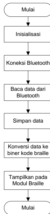
Gambar 9. Diagram alir program pada mikrokontroler
