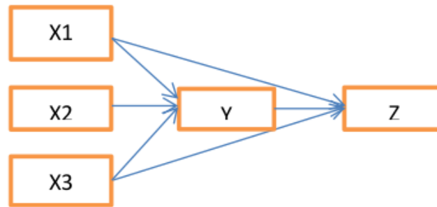
Gambar 3.2
