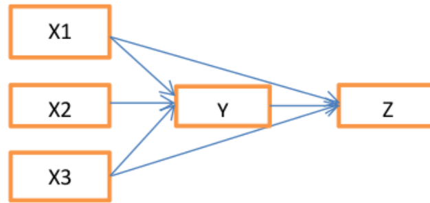
Gambar 3.1 Analisis Path
