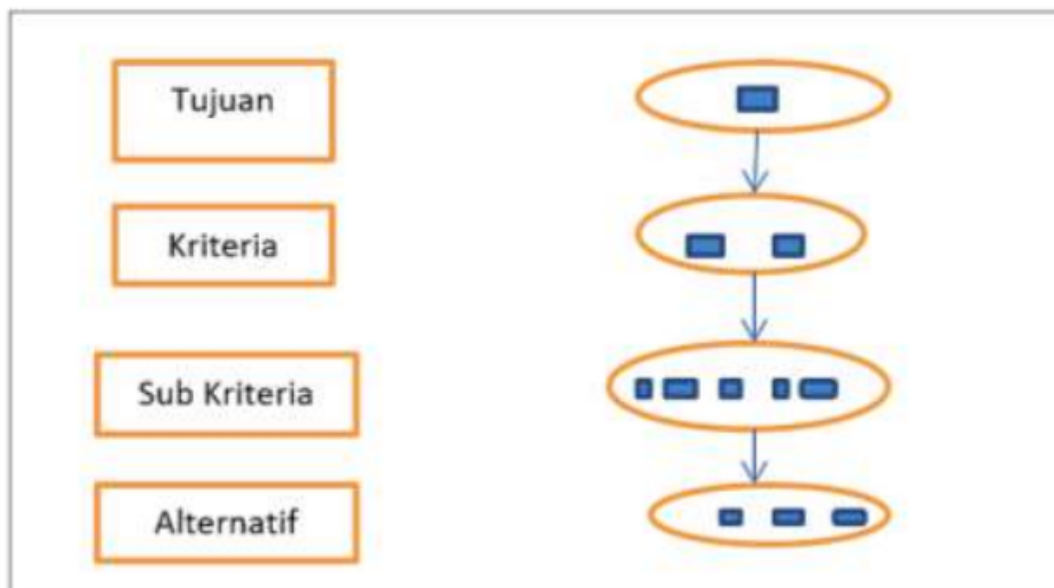
Gambar 7.2. Hierarki
