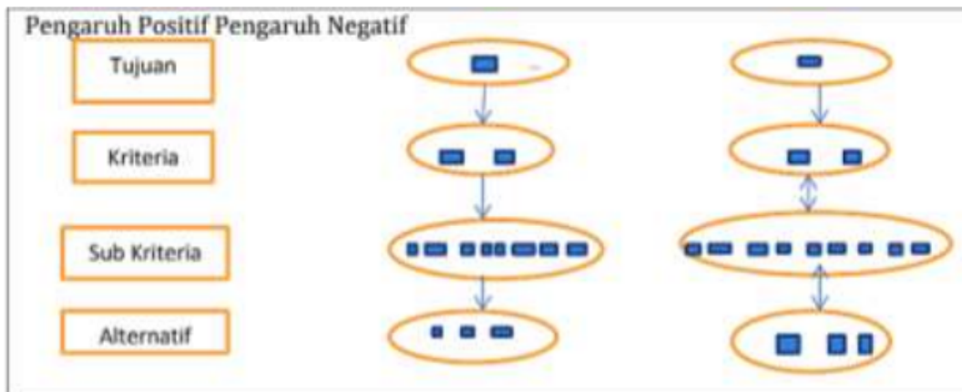
Gambar 7.4.
