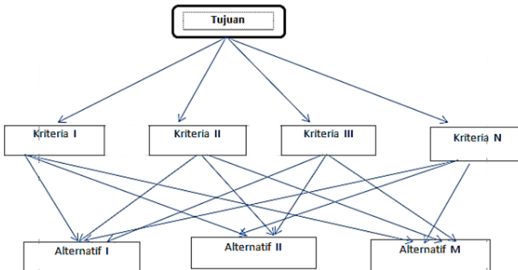
Gambar 6.1 Struktur Hierarki
