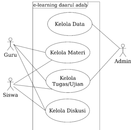
Gambar 2. Usecase diagram yang diusulkan
