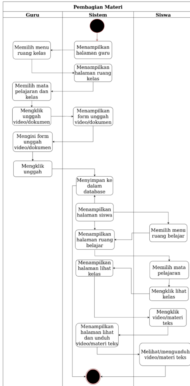
Gambar 3 Activity diagram pembagian materi
