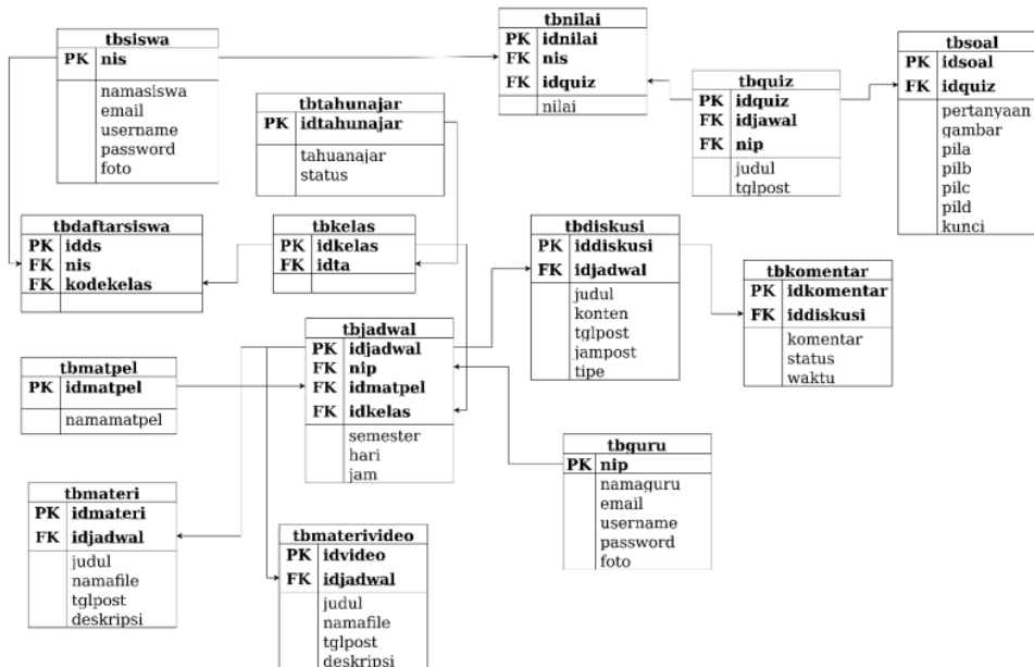
Gambar 5. relasi tabel
