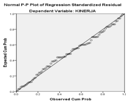
Gambar 3. Uji Normalitas
