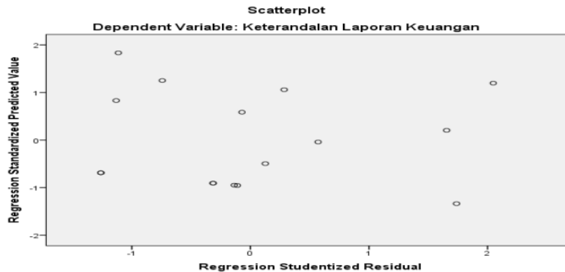
Gambar 2 Grafik Scatterplot
