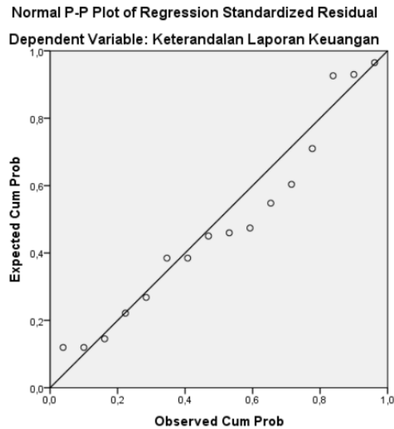
Gambar 1 Grafik Normalitas
