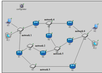
Gambar 3. Topologi non Optimasi
