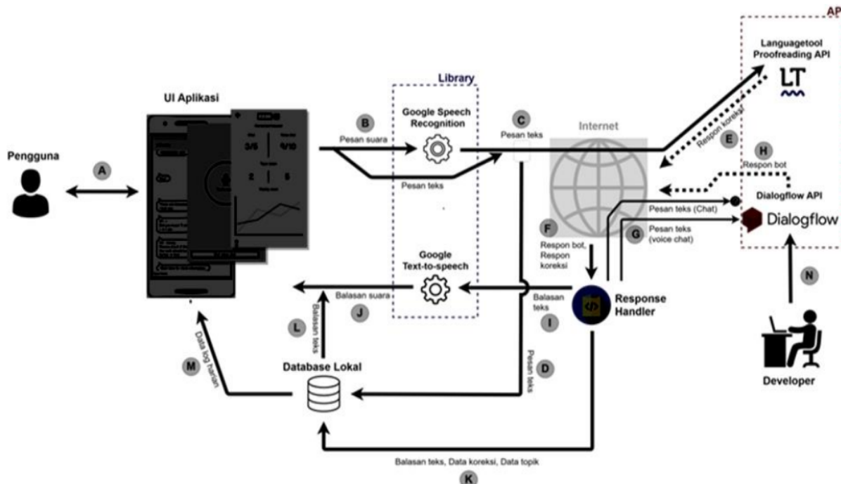
Gambar 4. Deskripsi Sistem Yang Dibangun
