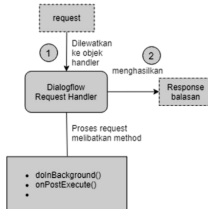
Gambar 11. Proses Request pada Dialogflow
