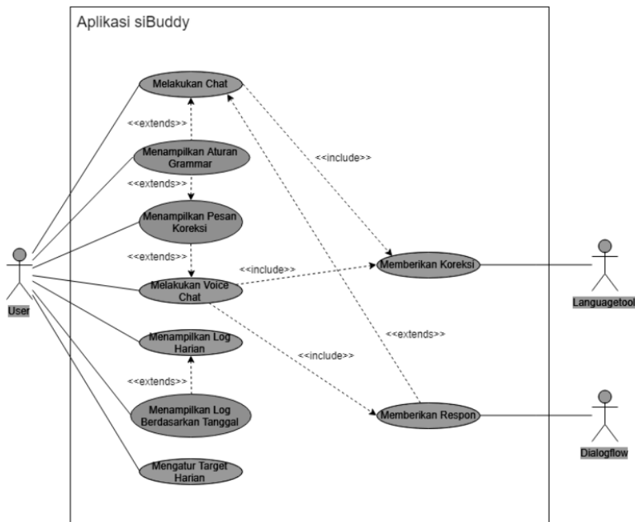
Gambar 12. Diagram Use Case Aplikasi Chatbot
