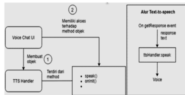
Gambar 8. TTS Handler dan Alur Text-To-Speech
