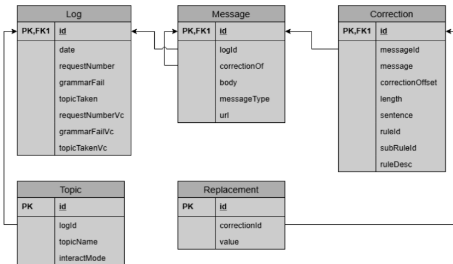
Gambar 13. Skema Relasi Tabel Aplikasi Chatbot
