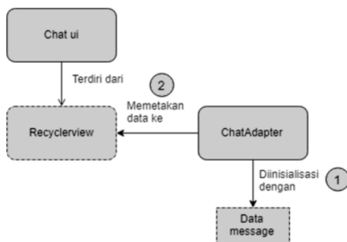
Gambar 6. Chat UI dan Chat Adapter
