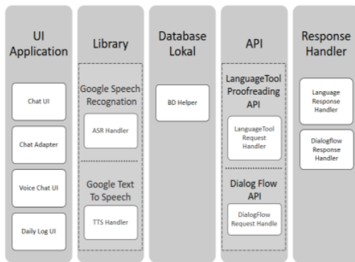
Gambar 5. Arsitektur Sistem
