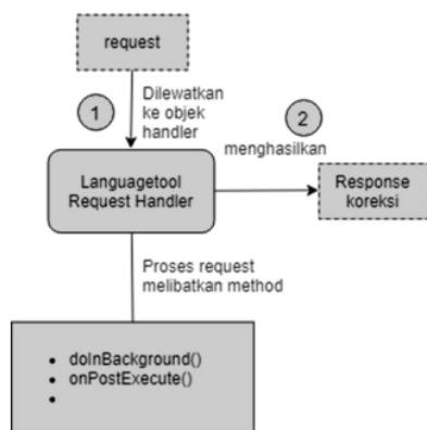
Gambar 10. Proses Request pada Languagetool
