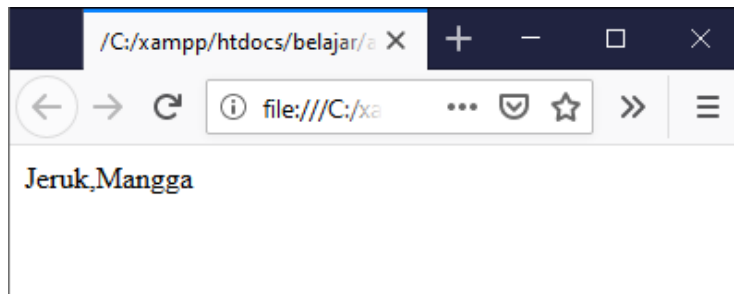
Gambar 12.5.Hasil Fungsi Slice
