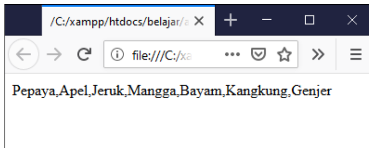
Gambar 12.12. Menggabung Array
