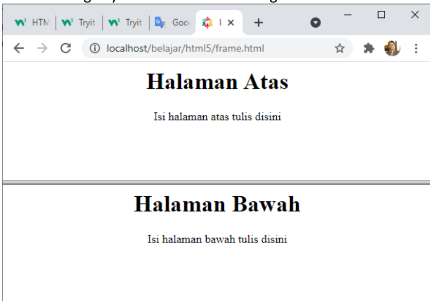
Gambar 7.1. Frameset 2 Baris
