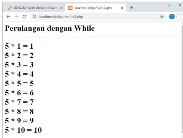
Gambar 6.3.Menampilkan Perkalian
