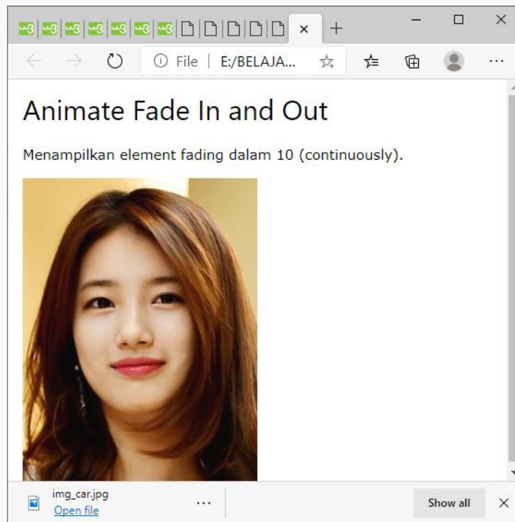
Gambar 12.7. Animate-fade
