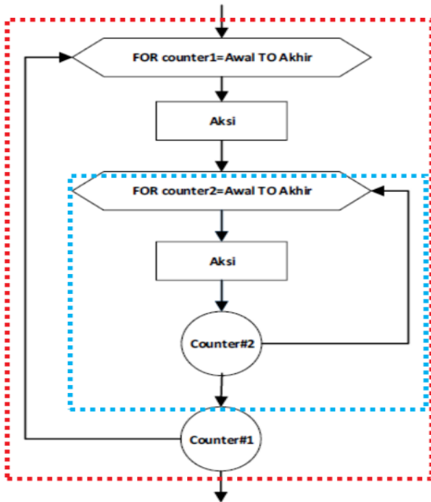
Gambar 3.8. Flow Chart Perulangan for dalam for
