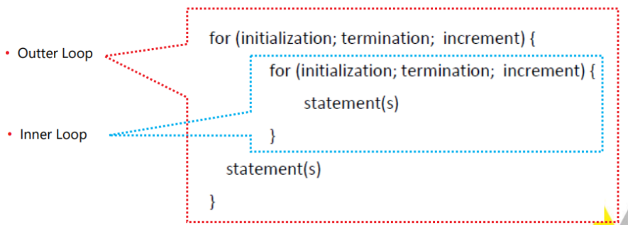
Gambar 3.7. Outer Loop dan Inner Loop
