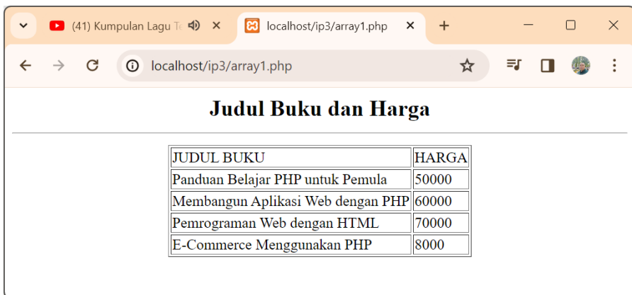
Gambar 3.6. Menampilkan array dengan perulangan for
