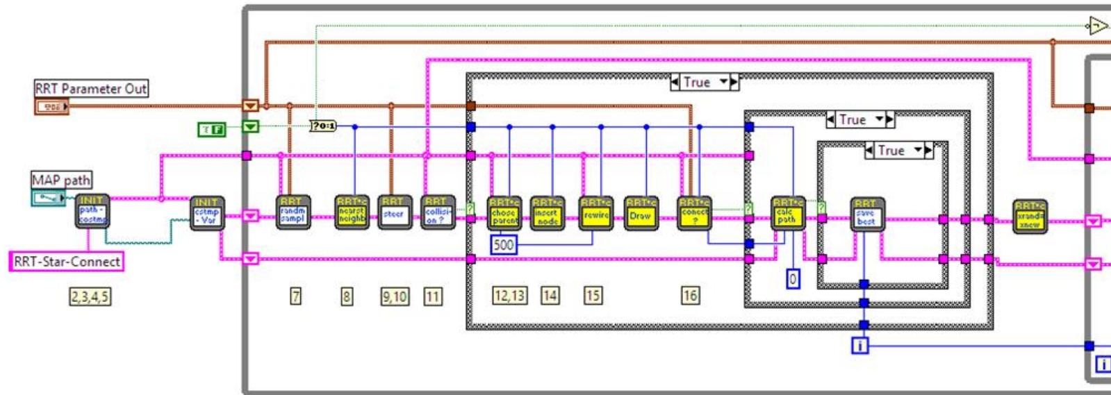
Gambar 8. Sebagian block diagram algoritma RRT*-Connect yang dibuat dengan library ini. Nomor dalam kotak kuning menunjukkan proses yang dijelaskan pada Algoritma 3 Gambar 3.
