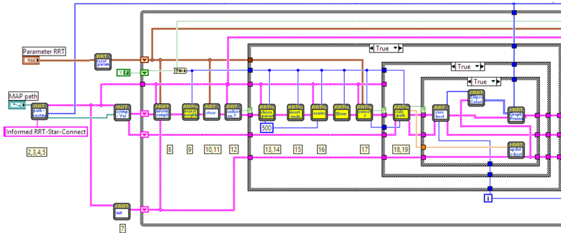
Gambar 10. Sebagian block diagram algoritma Informed RRT*-Connect yang dibuat dengan library ini. Nomor dalam kotak kuning menunjukkan proses yang dijelaskan pada Algoritma 5 Gambar 5.
