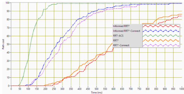
Gambar 24. Tools untuk analisis III: performansi dari suatu algoritma dapat divisualisasikan dalam bentuk grafik kecepatan konvergensi
