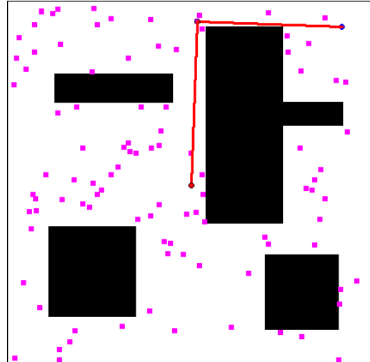
Gambar 20. Visualisasi contoh jalur lengkap dari algoritma PRM
