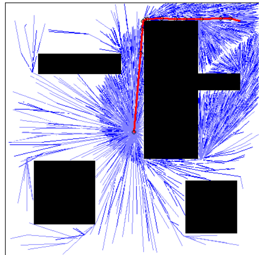
Gambar 17. Visualisasi contoh jalur lengkap dari algoritma RRT*-Connect
