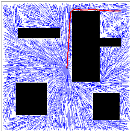
Gambar 15. Contoh jalur lengkap dari algoritma RRT* setelah melakukan iterasi sebanyak 9721.
