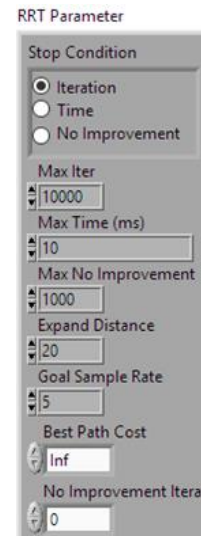
Gambar 26. Contoh front panel LabVIEW yang disediakan untuk mengubah parameter dari algoritma RRT*.
