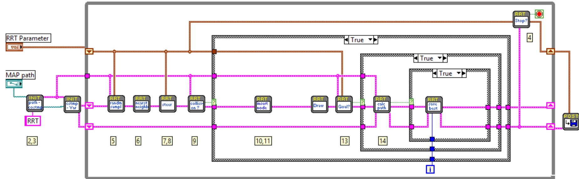
Gambar 6. Block diagram algoritma RRT yang dibuat dengan library ini. Nomor dalam kotak kuning menunjukkan proses yang dijelaskan pada Algoritma 1 Gambar 1.
