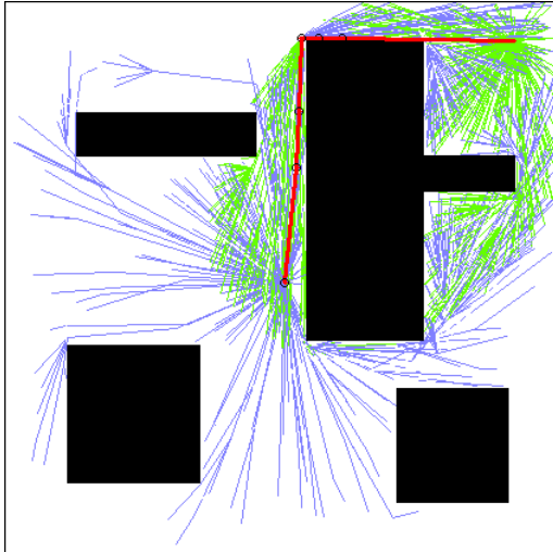
Gambar 18. Visualisasi contoh jalur lengkap dari algoritma Informed RRT*-Connect
