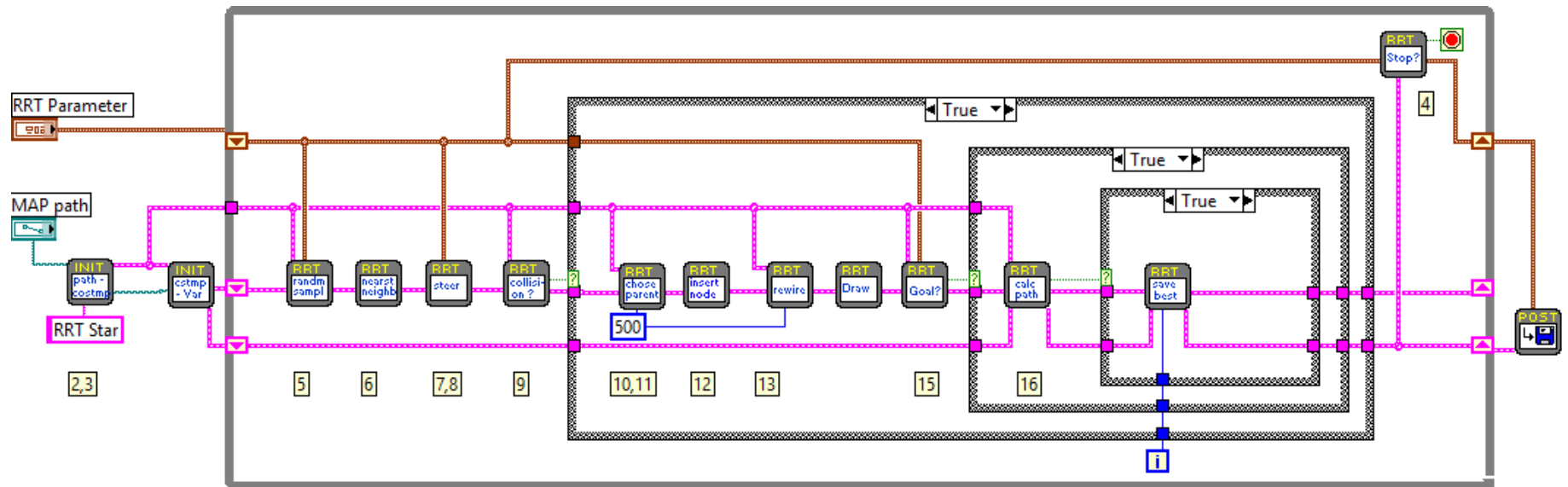
Gambar 7. Block diagram algoritma RRT* yang dibuat dengan library ini. Nomor dalam kotak kuning menunjukkan proses yang dijelaskan pada Algoritma 2 Gambar 2.
