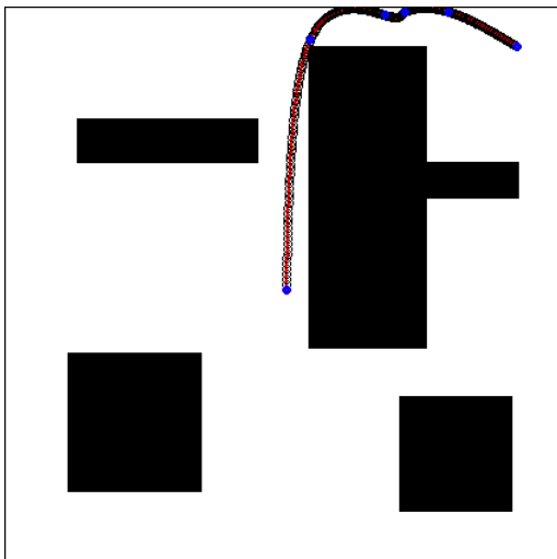
Gambar 23. Visualisasi jalur lengkap yang diperoleh algoritma perencanaan jalur berbasis PSO
