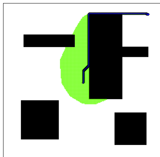
Gambar 21. Visualisasi contoh jalur lengkap dari algoritma A*
