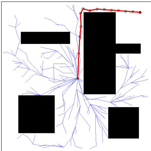
Gambar 19. Visualisasi contoh jalur lengkap dari algoritma RRT-ACS
