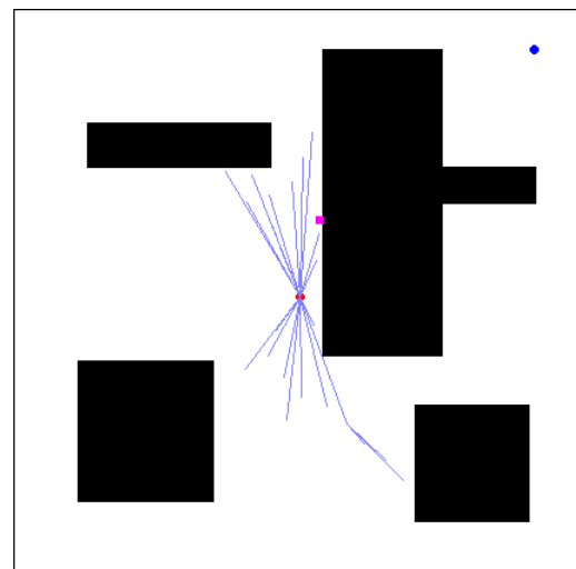
Gambar 13. Contoh Visualisasi dari pohon pencarian RRT*. Cabang baru dari pohon pencarian menuju node acak berwarna pink
