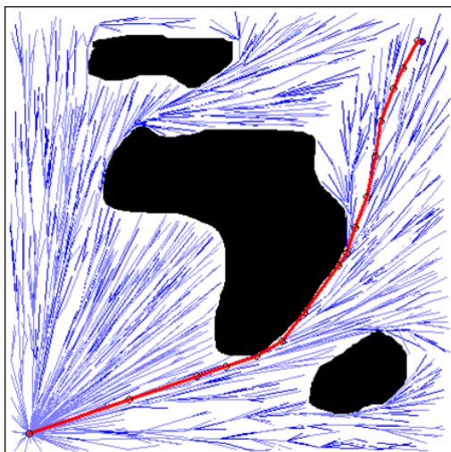
Gambar 25. Algoritma perencanaan jalur yang dibuat menggunakan library ini, bahkan dapat diimplementasikan pada lingkungan dengan obstacle berbentuk kurva
