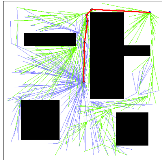
Gambar 16. Visualisasi jalur lengkap yang diperoleh algoritma RRT*-Connect
