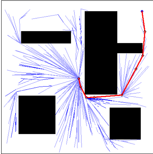
Gambar 14. Garis berwarna merah tebal adalah contoh jalur lengkap dari node awal ke node tujuan.
