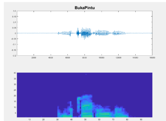
Gambar 11 Bentuk speech waveform dan speech spectrogram perintah ‘Buka Pintu’ pada intensitas background noise 24dB
