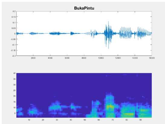
Gambar 23 Bentuk speech waveform dan speech spectrogram perintah ‘Buka Pintu’ pada intensitas background noise 52dB
