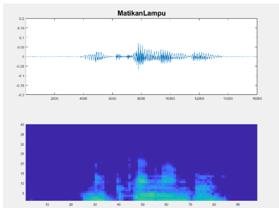
Gambar 9 Bentuk speech waveform dan speech spectrogram perintah ‘Matikan Lampu’ pada intensitas background noise 24dB
