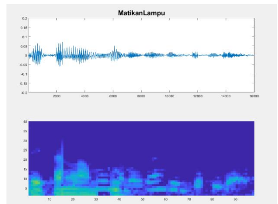
Gambar 21 Bentuk speech waveform dan speech spectrogram perintah ‘Matikan Lampu’ pada intensitas background noise 52dB
