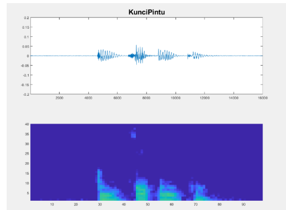
Gambar 10 Bentuk speech waveform dan speech spectrogram perintah ‘Kunci Pintu’ pada intensitas background noise 24dB
