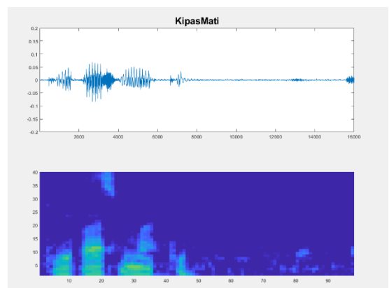
Gambar 19 Bentuk speech waveform dan speech spectrogram perintah ‘Kipas Mati’ pada intensitas background noise 42dB
