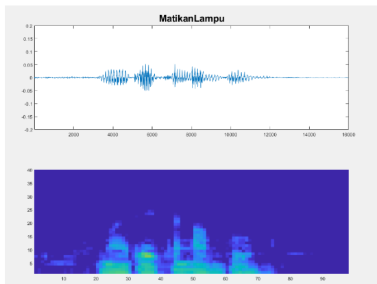
Gambar 15 Bentuk speech waveform dan speech spectrogram perintah ‘Matikan Lampu’ pada intensitas background noise 42dB
