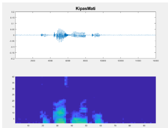
Gambar 13 Bentuk speech waveform dan speech spectrogram perintah 'Kipas Mati' pada intensitas background noise 24dB
