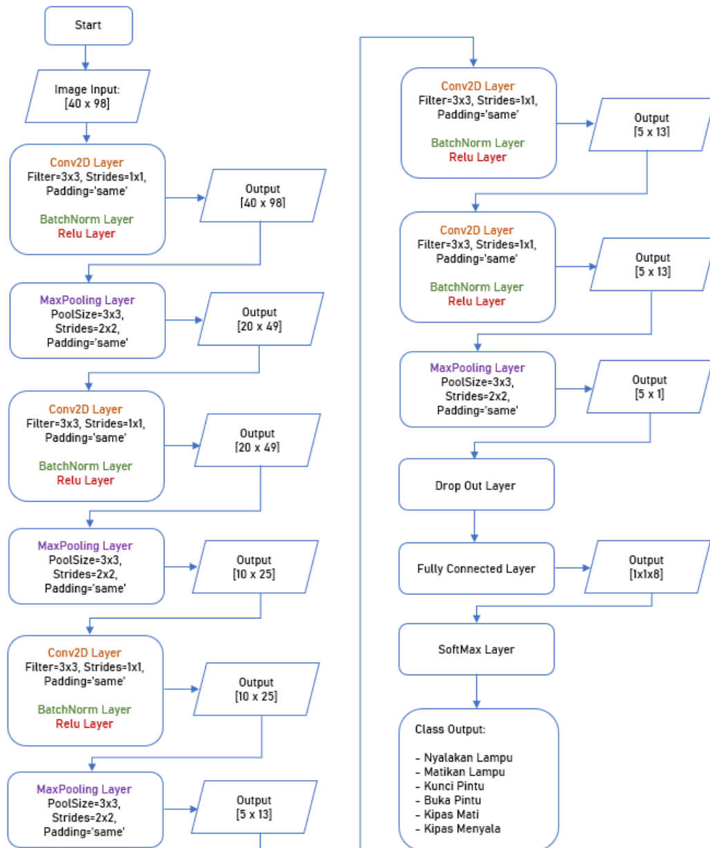
Gambar 5 Flowchart proses klasifikasi
