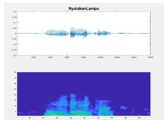
Gambar 14 Bentuk speech waveform dan speech spectrogram perintah 'Nyalakan Lampu' pada intensitas background noise 42dB
