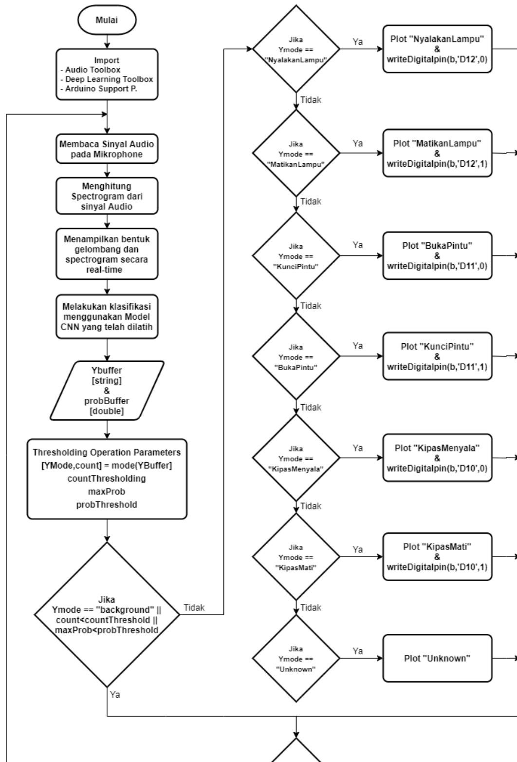
Gambar 7 Flowchart pendeteksian perintah suara untuk mengendalikan perangkat elektronik
