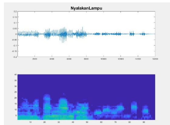
Gambar 20 Bentuk speech waveform dan speech spectrogram perintah ‘Nyalakan Lampu’ pada intensitas background noise 52dB
