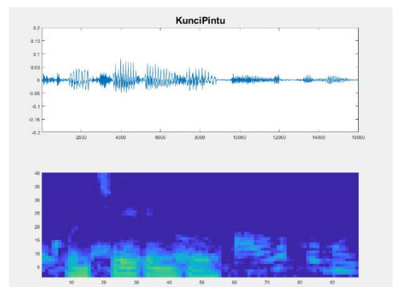
Gambar 22 Bentuk speech waveform dan speech spectrogram perintah ‘Kunci Pintu’ pada intensitas background noise 52dB
