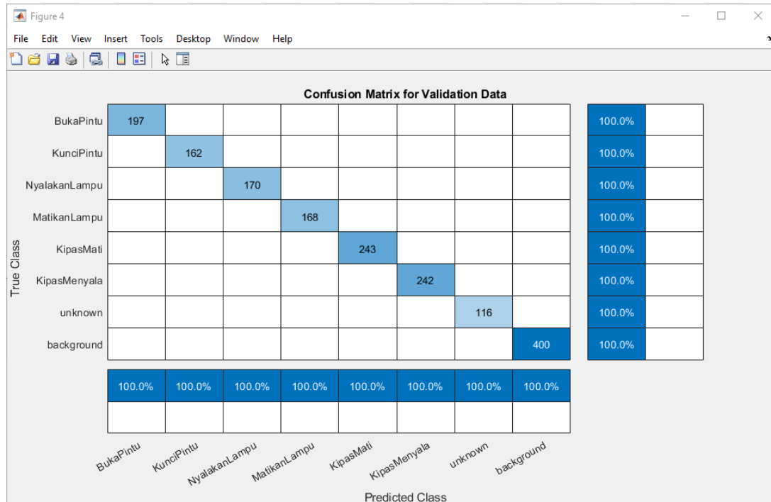
Gambar 6 Evaluasi model CNN
