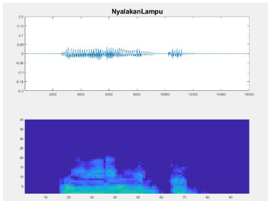
Gambar 8 Bentuk speech waveform dan speech spectrogram perintah ‘Nyalakan Lampu’ pada intensitas background noise 24dB
