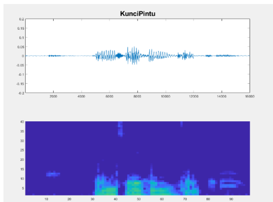
Gambar 16 Bentuk speech waveform dan speech spectrogram perintah ‘Kunci Pintu’ pada intensitas background noise 42dB
