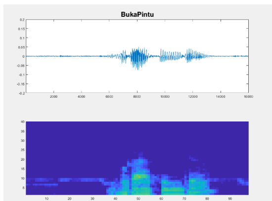
Gambar 17 Bentuk speech waveform dan speech spectrogram perintah ‘Buka Pintu’ pada intensitas background noise 42dB
