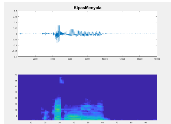
Gambar 12 Bentuk speech waveform dan speech spectrogram perintah ‘Kipas Menyala’ pada intensitas background noise 24dB
