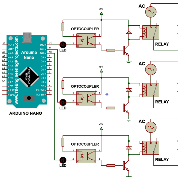
Gambar 2 Diagram skematik sistem
