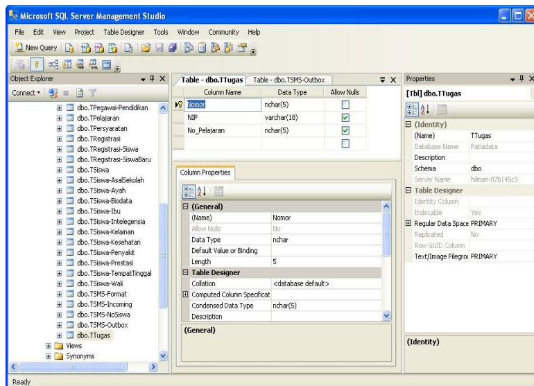
Gambar 9. Database Tugas
