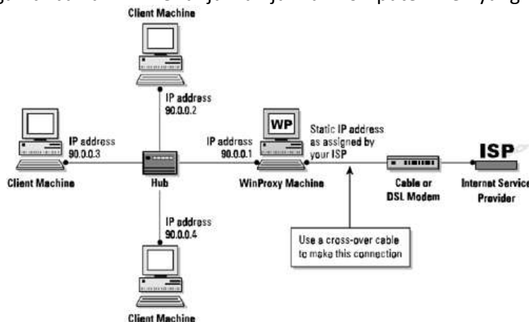
Gambar 3.5 Topografi LAN Menggunakan Kabel / Model DSL
