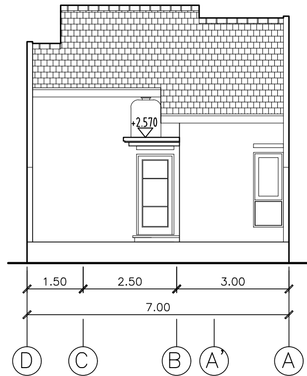
TAMPAK BELAKANG SKALA 1: 100
