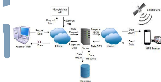
Gambar 4. Konsep Arsitektur Sistem
