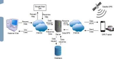
Gambar 4. Konsep Arsitektur Sistem
