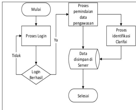
Gambar 3 Diagram alir proses pengawasan pada smartphone target
