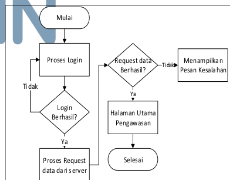
Gambar 2 Diagram alir proses pengawasan penggunaan smartphone
