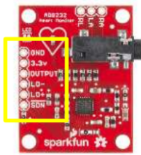
Fig. 8. Pin label on AD8232
