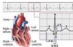
Fig. 1. ECG Waves
