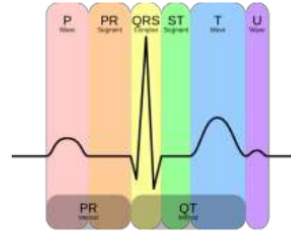
Fig. 5. QRS waves
