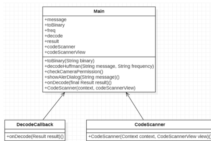
Gambar 8. Class diagram aplikasi pemindai
