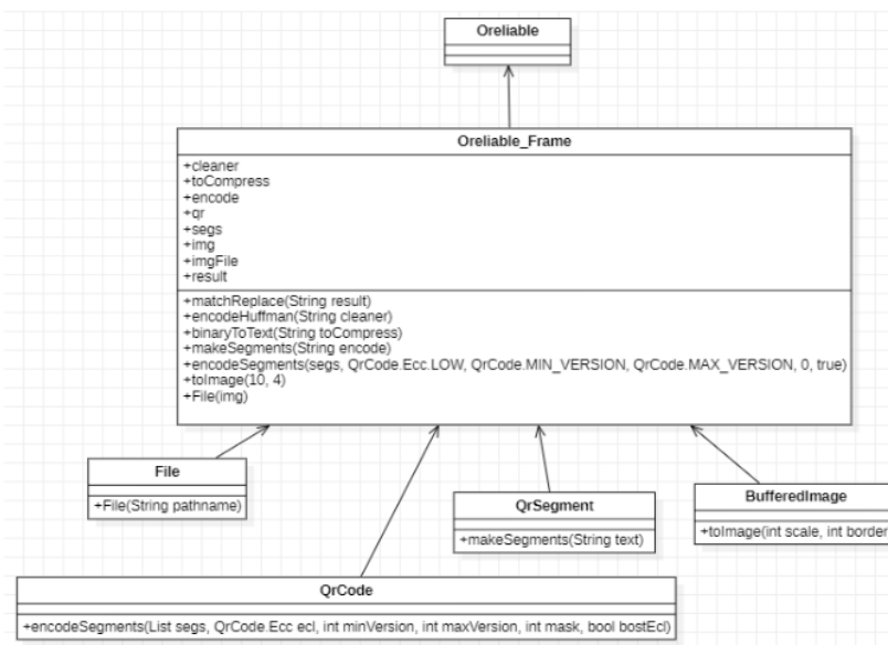
Gambar 7. Class diagram aplikasi generator
