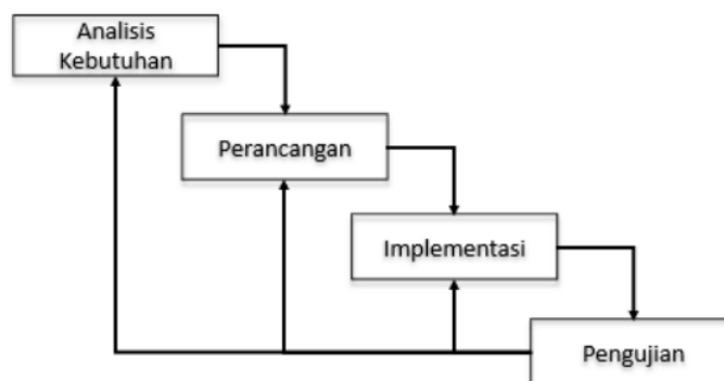
Gambar 2. Tahapan penelitian pada pengembangan aplikasi [20].
