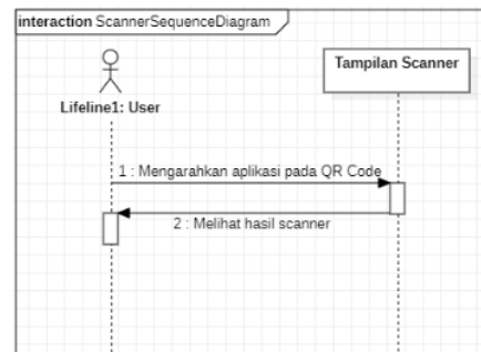
Gambar 6. Sequence diagram aplikasi pemindai kode QR
