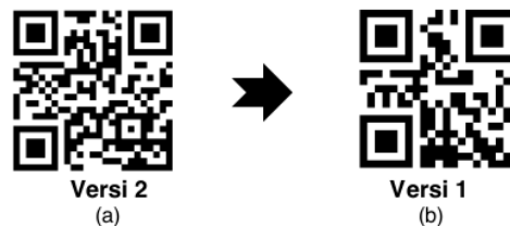
Gambar 13. Contoh kode QR, a) kode QR sebelum proses kompresi, b) kode QR setelah proses kompresi
