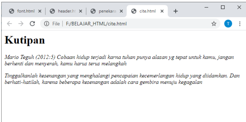
Gambar 2.15. Menampilkan kutipan
