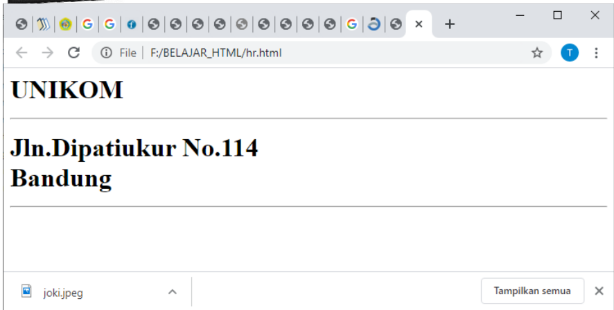
Gambar 2.17. Menggunakan BR
